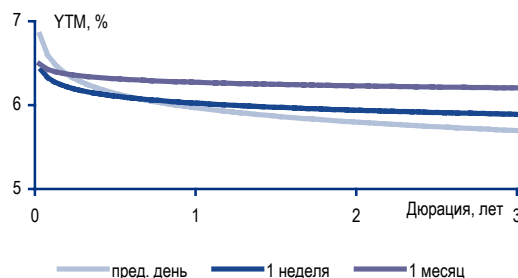
Изменение кривой NDF долл./руб. – LIBOR
